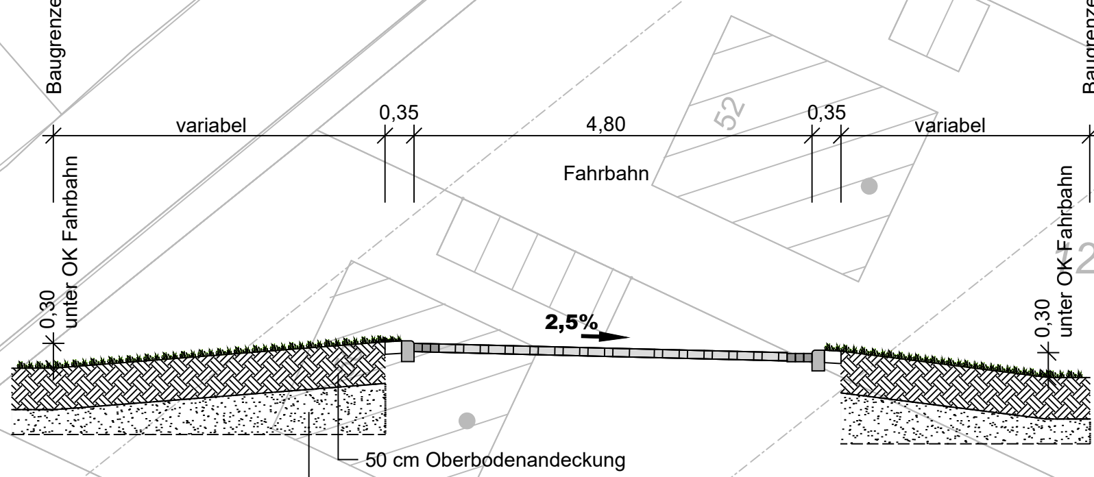
Systemschnitt D-D
