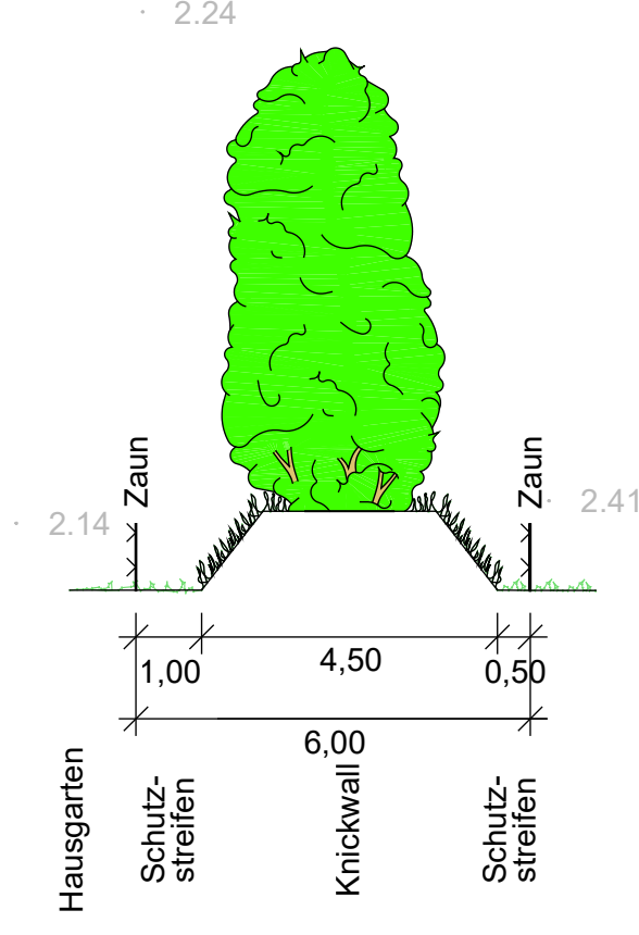
Schnitt C-C
